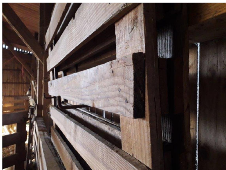
Photo : un système d’accroche des claies sur le bardage CP : CIIRPO
